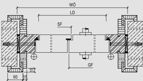
Detailzeichnung zu Bild 01
